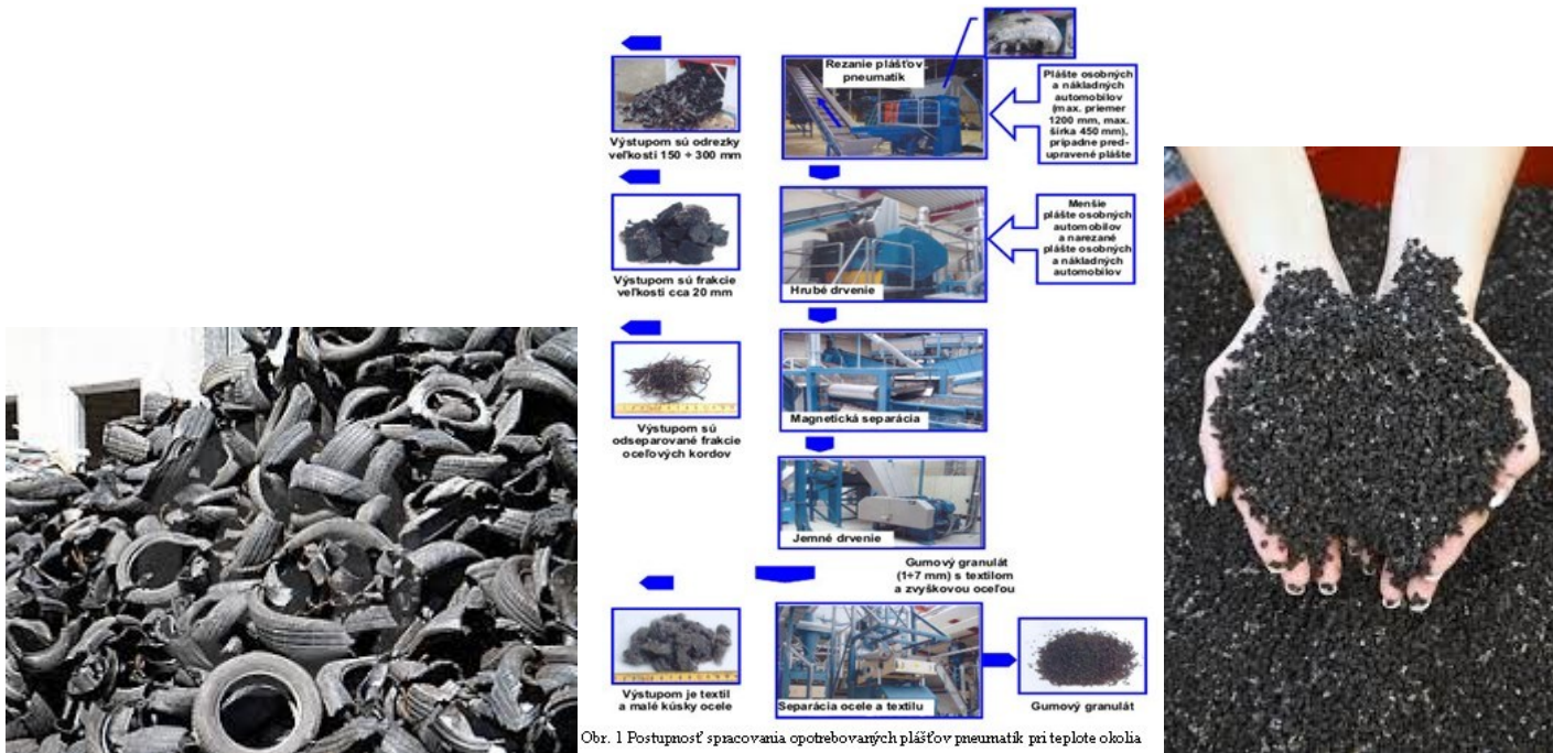
Obz. 1 Postupnosť spracovania opotrebovaných plášťov pneumatík pri teplote okolia
